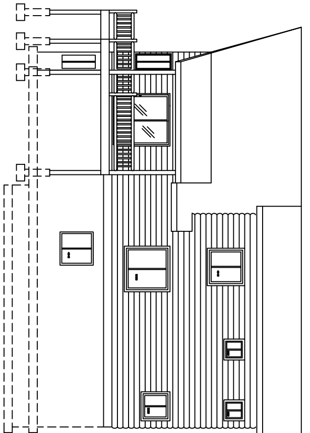
RIGHT ELEVATION
